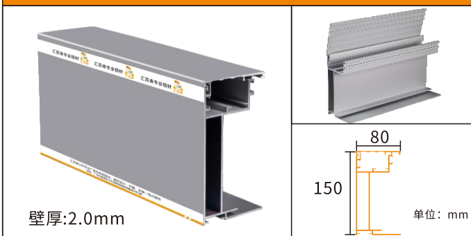
HBMA80-150工程拉布铝型材
