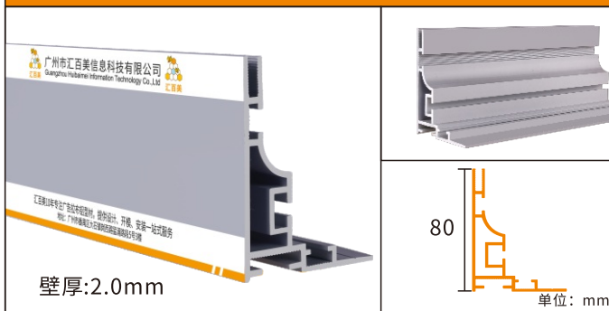
HBMCX-80卡布铝型材
