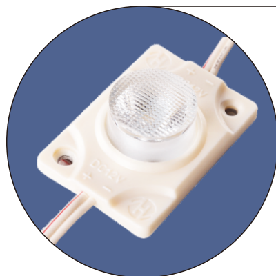
可调节大功率侧光源恒压防水 电 压：12V 光通量：200Lm 色 温：6000K-7000K 型 号：HBMH-CTF
