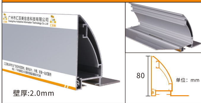
HBMB-80侧面开启拉布铝型材
