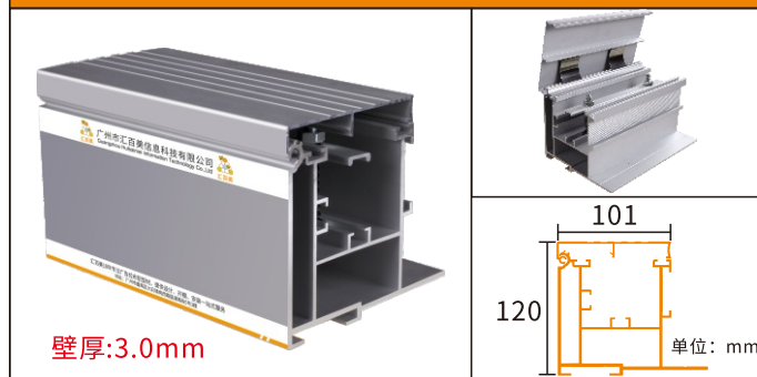
HBMAX-X-101-120工程加强加厚拉布铝型材
