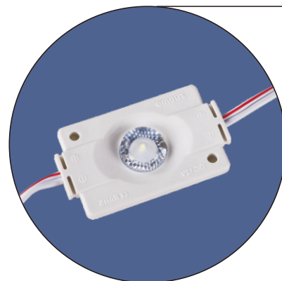
SMD3030单颗大功率 电 压：12V 光通量：168Lm 色 温：13000K-15000K 型 号：HBMGJ-CT-3030
