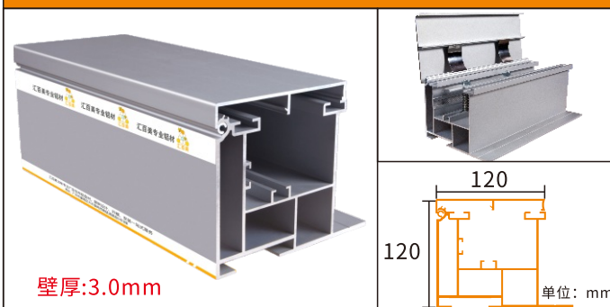
HBMAX-G-B-120-120工程加强加厚拉布铝型材
